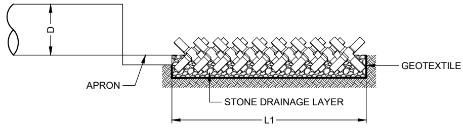
SECTION N.T.S.
